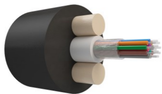
ДРОП-КРУГЛЫЙ С ЦЕНТРАЛЬНОЙ ТРУБКОЙ, УСИЛЕН СТЕКЛОПРУТКАМИ
