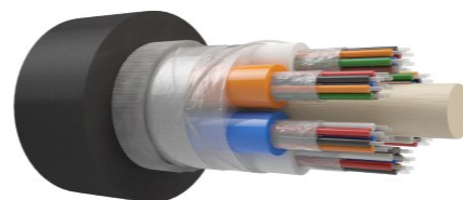
КАБЕЛЬ ОПТИЧЕСКИЙ ПОДВЕСНОЙ САМОНЕСУЩИЙ, МНОГОМОДУЛЬНЫЙ, АРМИРОВАННЫЙ СТЕКЛОНИТЯМИ
