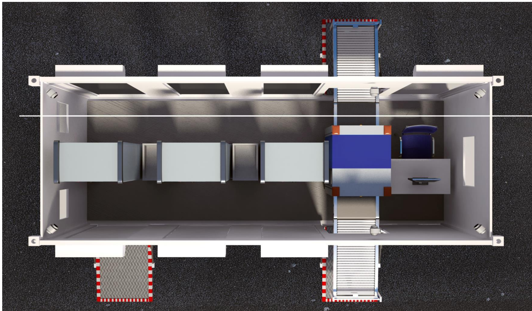
МПД «ВС РУБЕЖ-3/1» (вид сверху)
