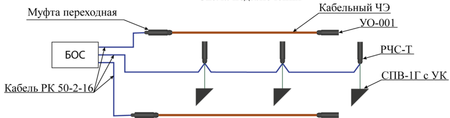
Схема подключения
