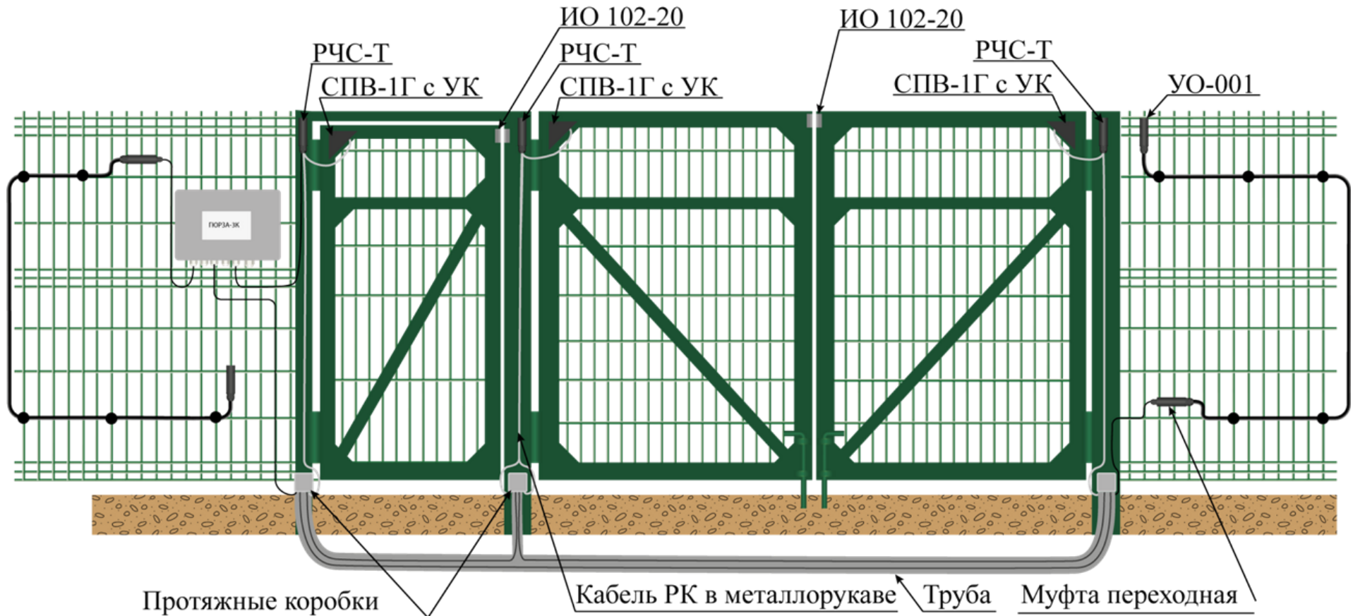
Схема подключения
